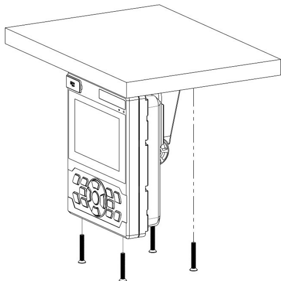
نصب بر روی سقف
